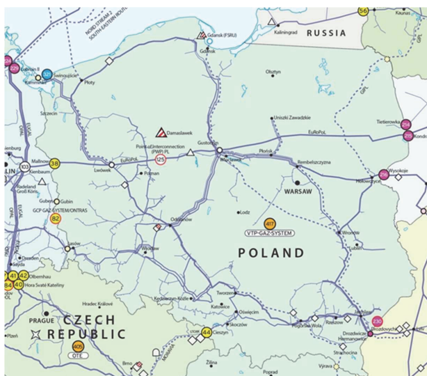
Σχήμα 17: Το Σύστημα Φυσικού Αερίου της Πολωνίας
